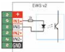
Schéma de l'optocoupleur d'entrée EWS
